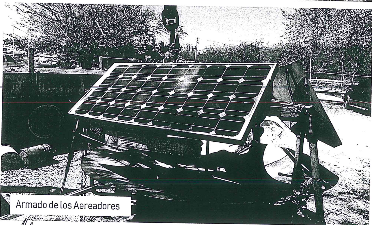
Armado de los Aereadores
